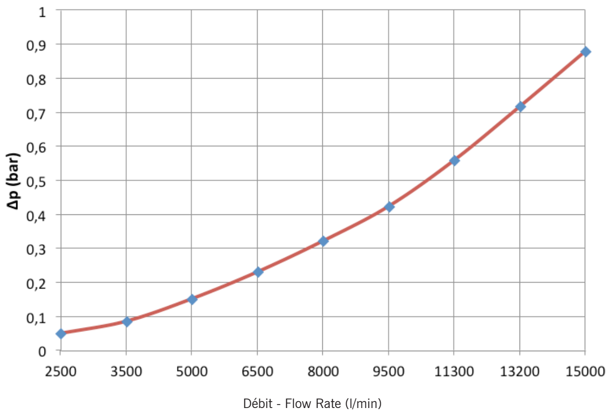
PROPORTIONNEUR Ø12" / MIXER Ø12"
