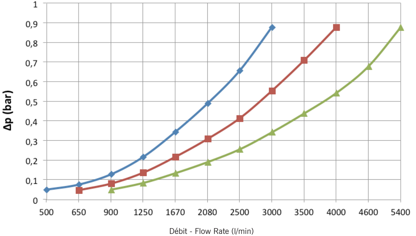
PROPORTIONNEUR Ø6" / MIXER Ø6"
