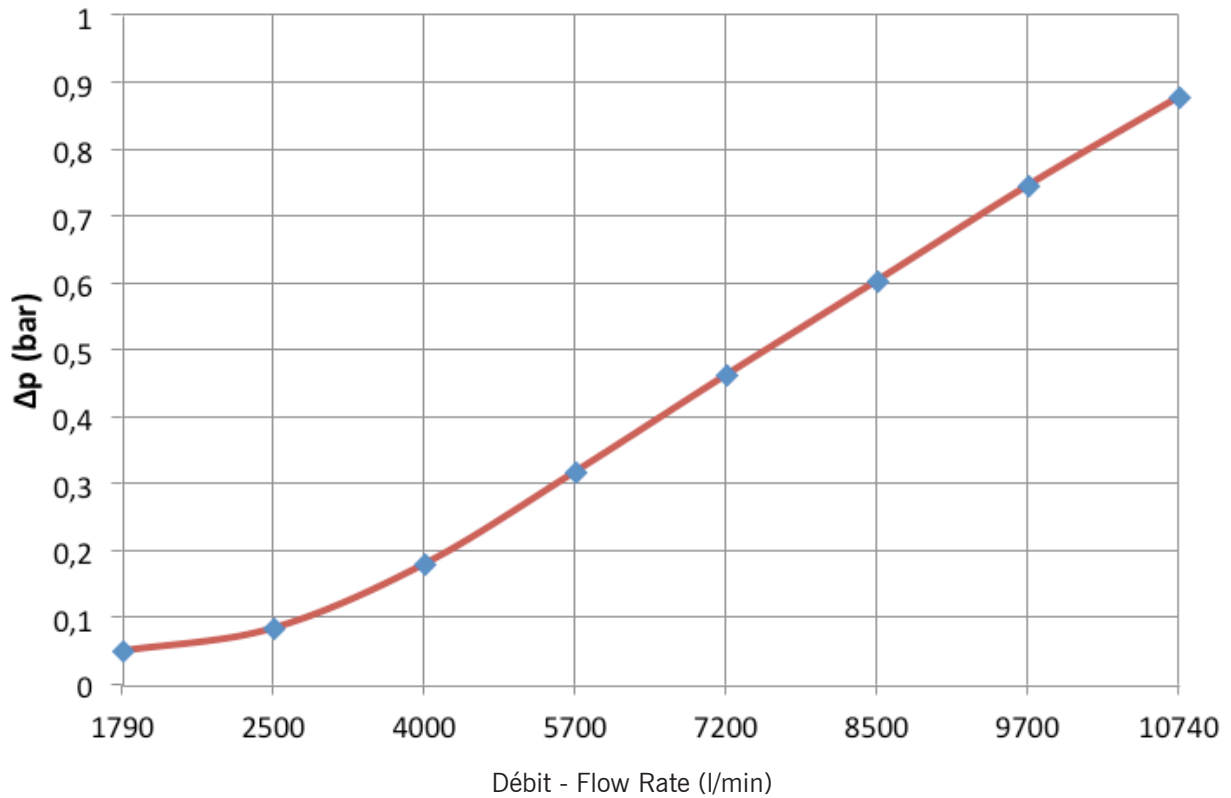
PROPORTIONNEUR Ø12" / MIXER Ø12"
