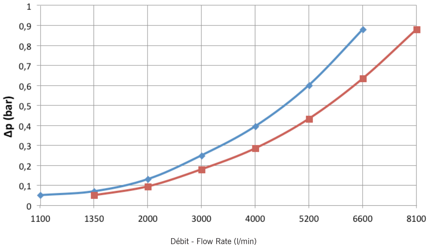
PROPORTIONNEUR Ø8" / MIXER Ø8"
