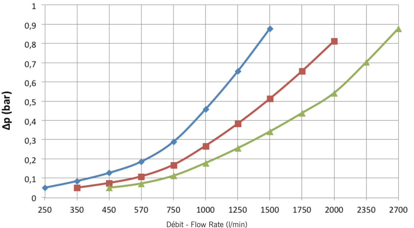
PROPORTIONNEUR Ø4" / MIXER Ø4"
